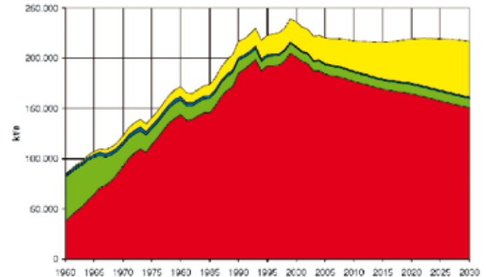
Abbildung: Kohlenstoffdioxidemissionen des Verkehrs nach Verkehrsträgern (TREMOT 2006)
